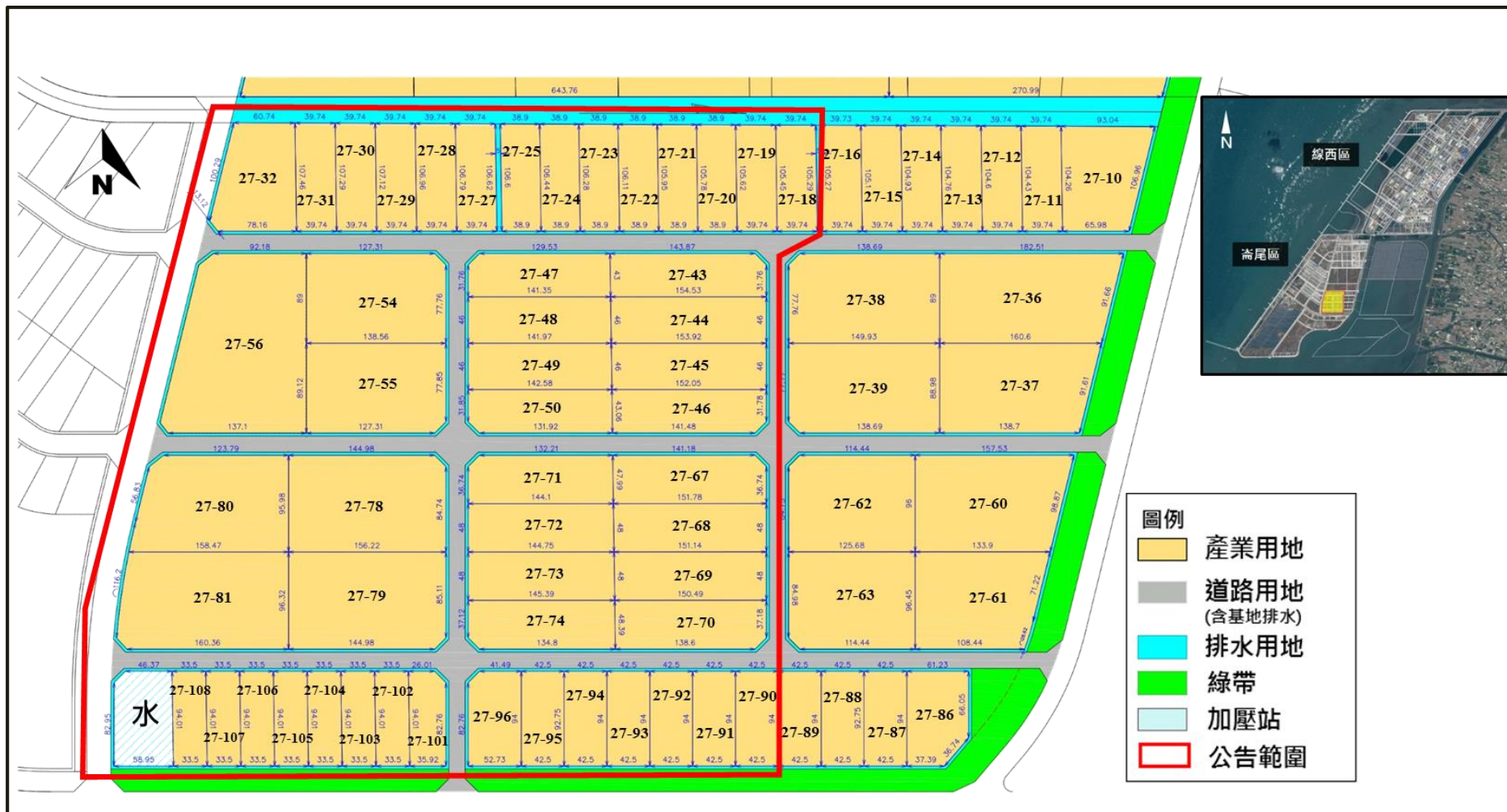
附圖2、彰濱工業區崙尾西一區四期產業用地(一)土地坵塊尺寸圖
